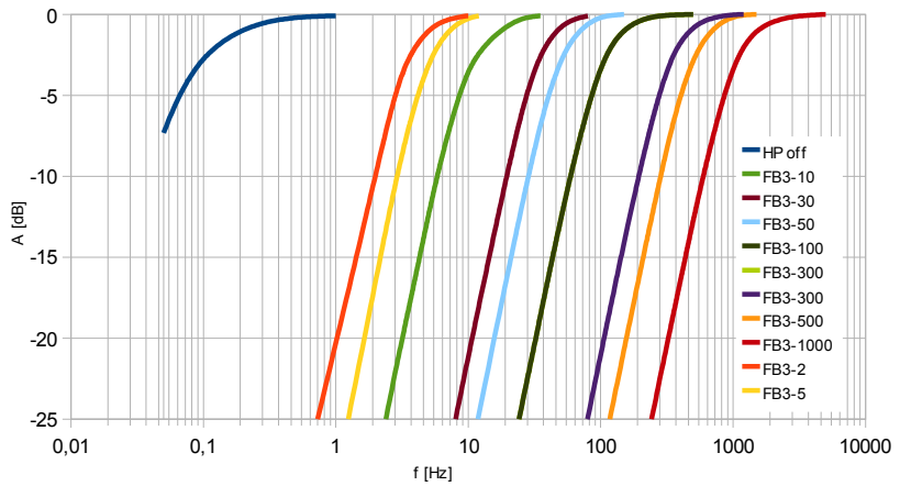
Bild 9: Amplitudenfrequenzgang des M208B mit den Hochpassfiltern FB3-...
